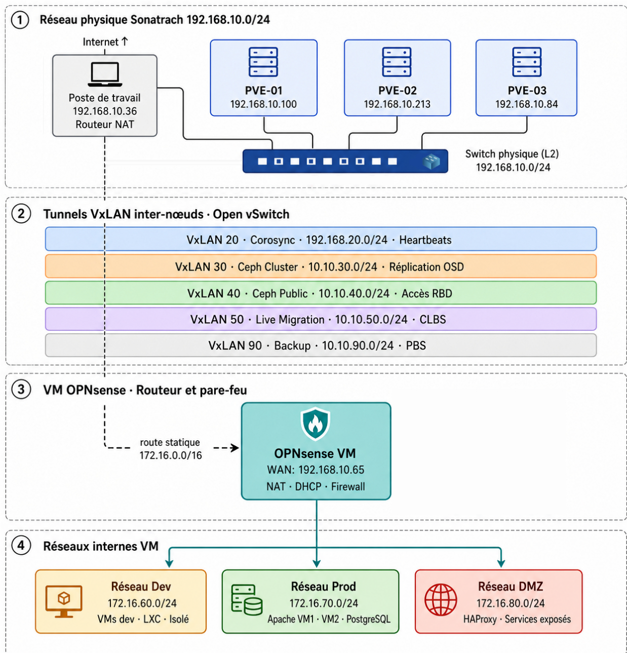
FIGURE III.4 – Topologie Réseau et Plan VxLAN
